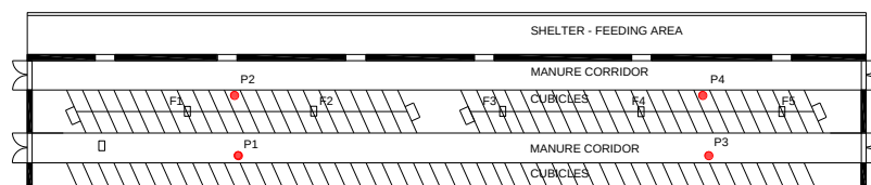
Obr. 1 Pôdorys objektu A s meracími bodmi P1 – P4 k meraniam koncentrácií plynov a bodmi merania parametrov mikroklimy 1 - 4
