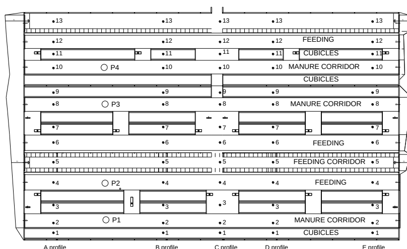
Obr. 2 Pôdorys objektu B s meracími bodmi P1 – P4 k meraniam koncentrácií plynov a bodmi merania parametrov mikroklimy 1 - 13
