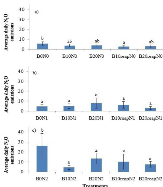
Obrázok 1. Priemerné emisie \text{N}_2\text{O} za skúmané obdobie z nehnojeného variantu N0 (a), hnojeného variantu N1 (b) a N2 (c) v kombinácií s biouhlím a bez neho.
